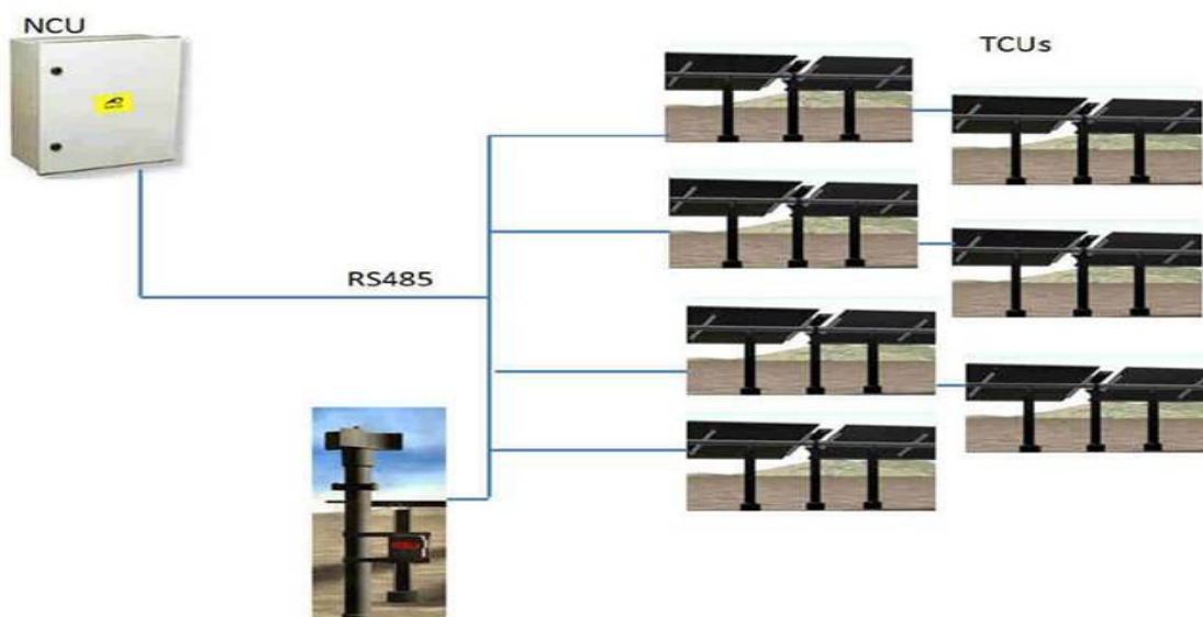
Imagen 12. Estación básica (NCU = Network Control Unit)
