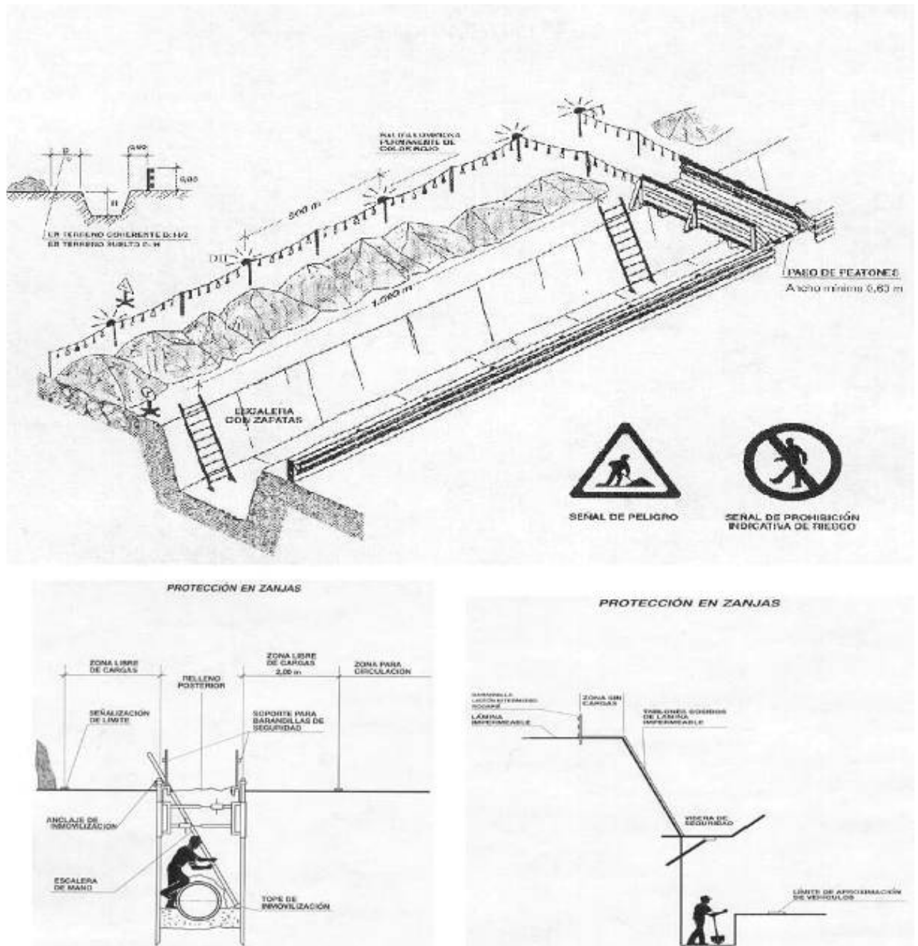
Figura 21: Protección, señalización y entibación de zanjas.
