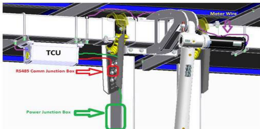
Imagen 11. Posición de la TCU (se puede alimentar de la red o puede ser autoalimentado)
