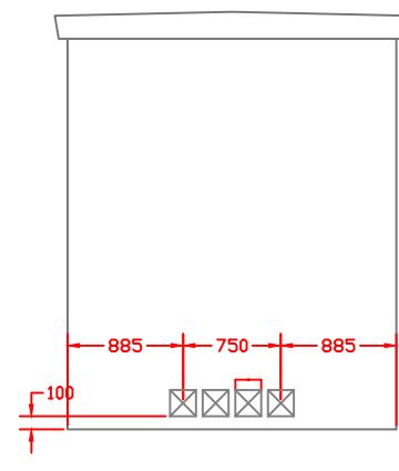
PERFIL DERECHO
