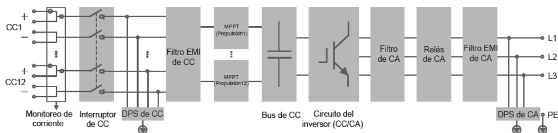
Imagen 6. Esquema conexiones Inversor.
