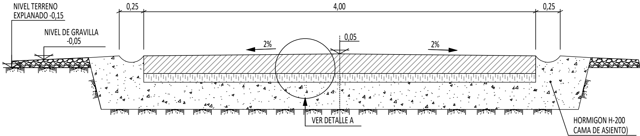
SECCION VIAL TIPO
