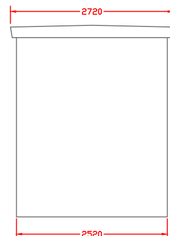
PERFIL IZQUIERDO
