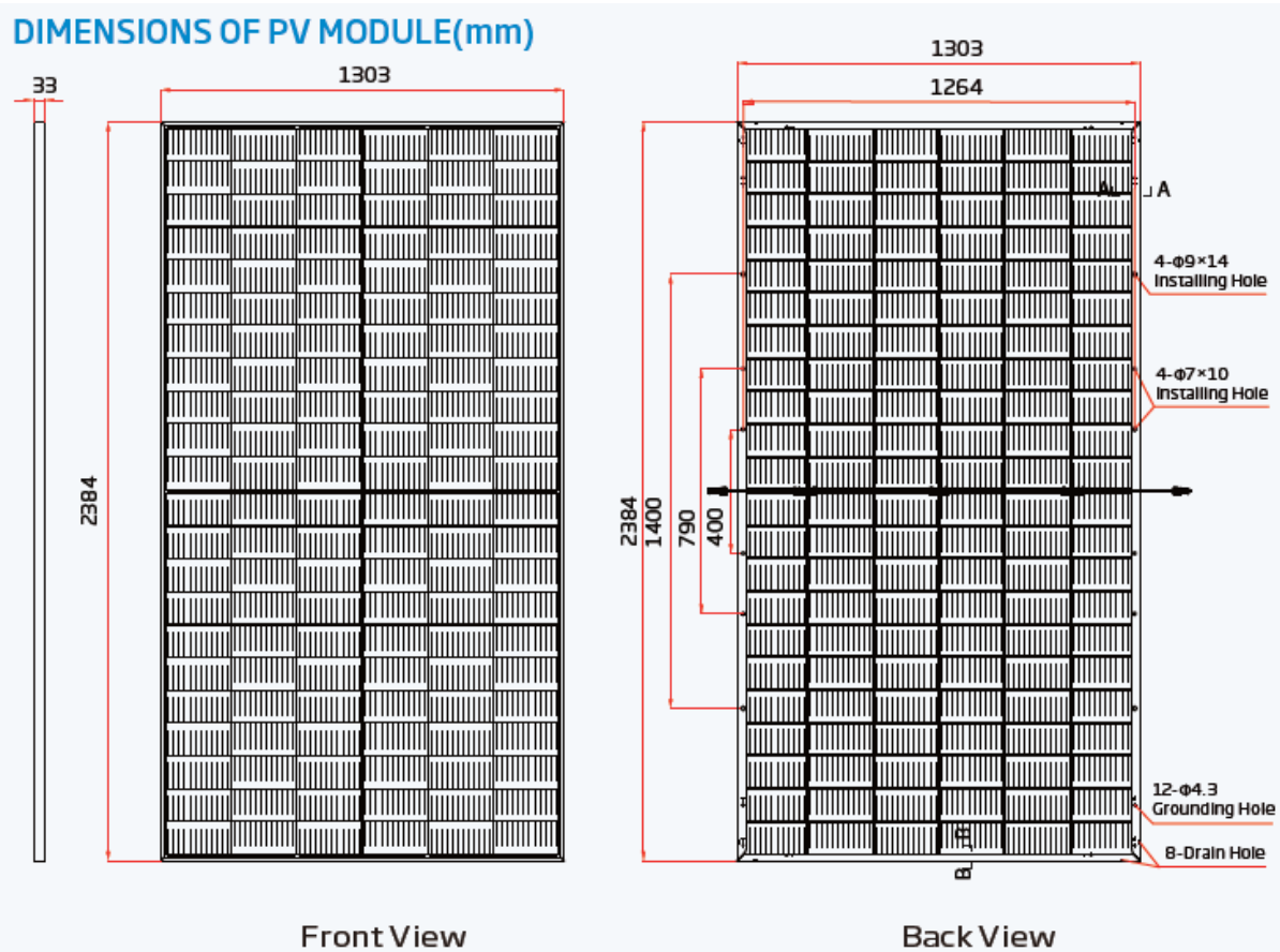
Imagen 4. Dimensiones físicas del módulo.
