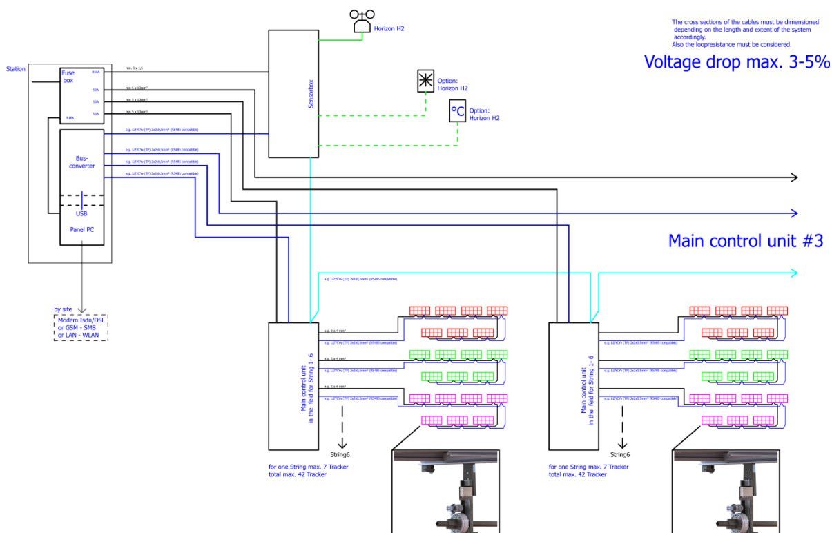
Imagen 10. Esquema de comunicaciones general.
