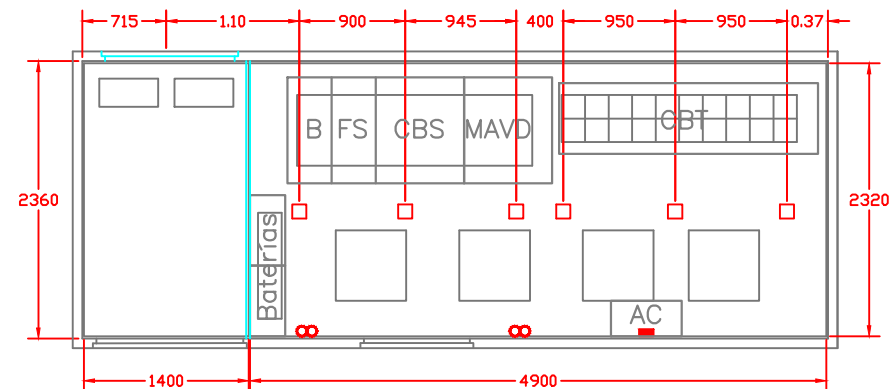
PERFIL IZQUIERDO
