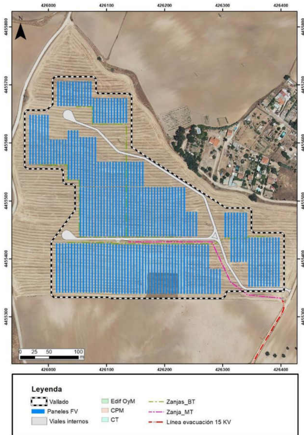
Figura 10. Detalle de la implantación de la planta fotovoltaica sobre ortofoto. Fuente: Elaboración propia a partir de datos del promotor.
