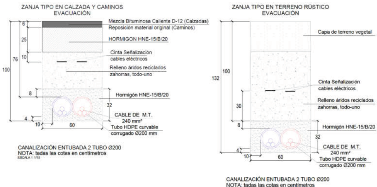
Figura 15. Detalle secciones tipo. Fuente: Proyecto de ejecución.
