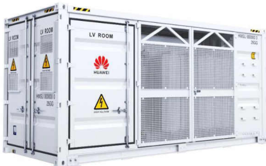
Figura 14. Centro de transformación Huawei STS6000H1. Fuente: Proyecto ejecución.
