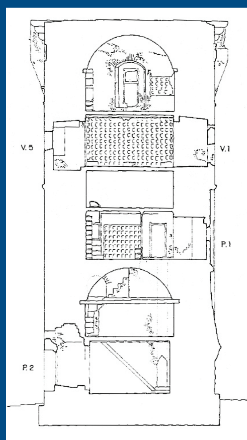
Alzado interior del edificio.
