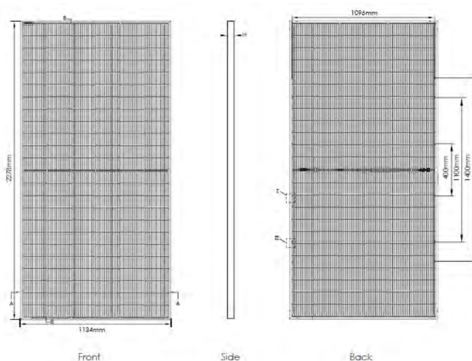
Ilustración 14. Módulo fotovoltaico
