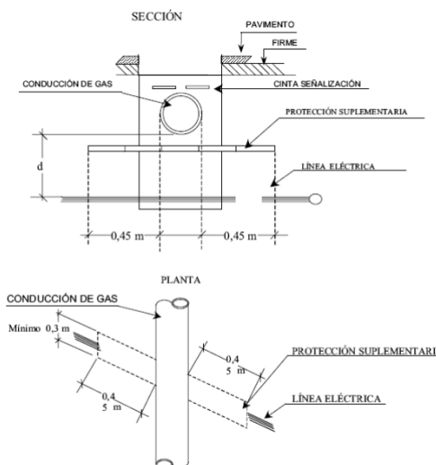
Ilustración 41. Detalles de cruzamiento y conducciones (ITC-LAT 06)
