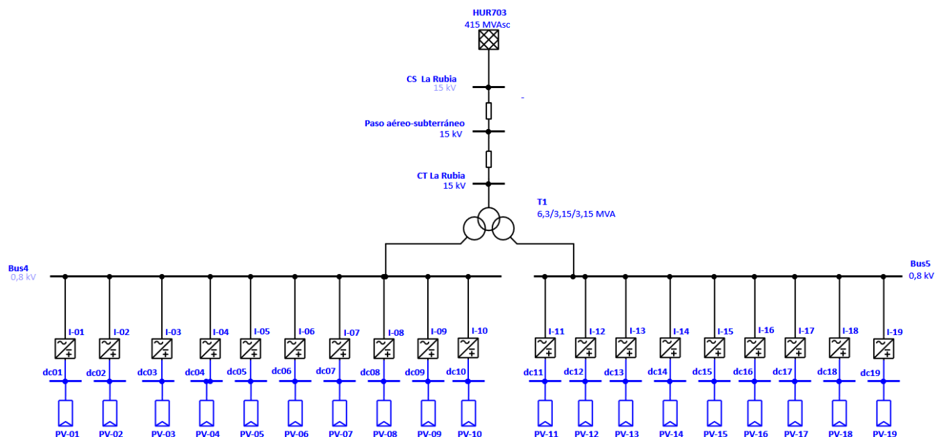
Ilustración 1. Modelo estudio cortocircuito
