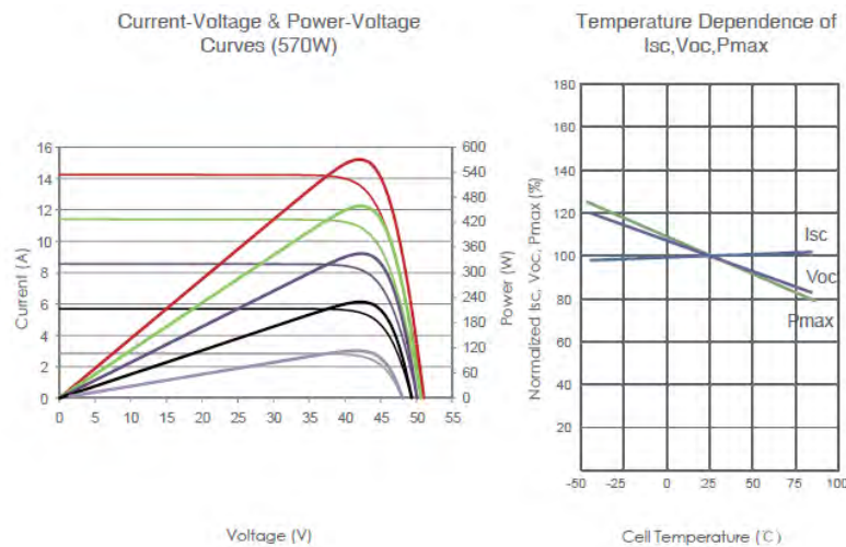
Ilustración 15. Curvas características
