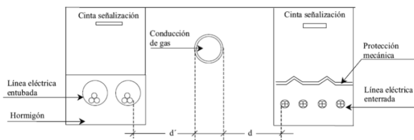
Ilustración 43. Detalles de paralelismo y conducciones (ITC-LAT 06)
