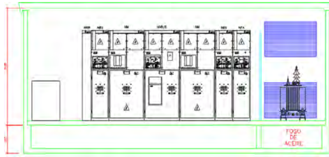
Ilustración 24. Sección CPM
