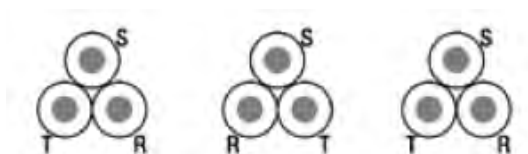
Ilustración 38. Colocación de cables en tresbolillo
