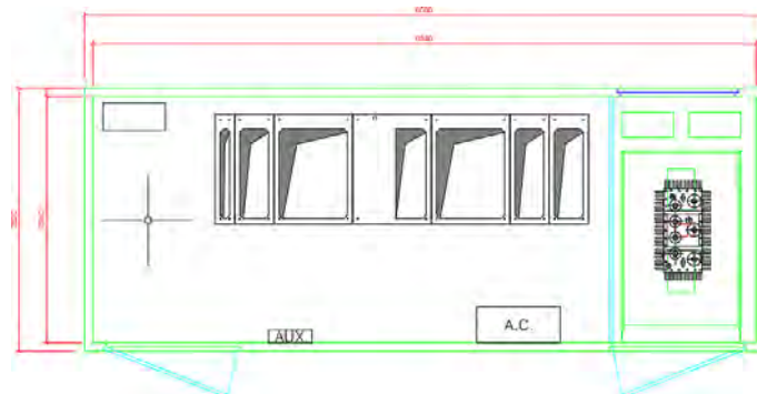
Ilustración 23. Planta CPM
