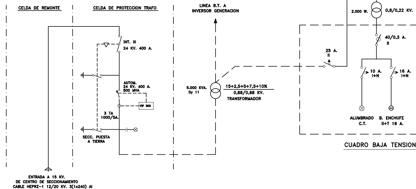
ESQUEMA UNIFILAR
