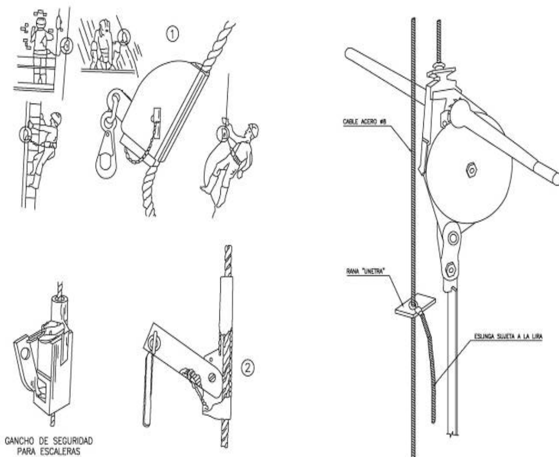
Figura 6: Anclajes móviles para cinturones.
