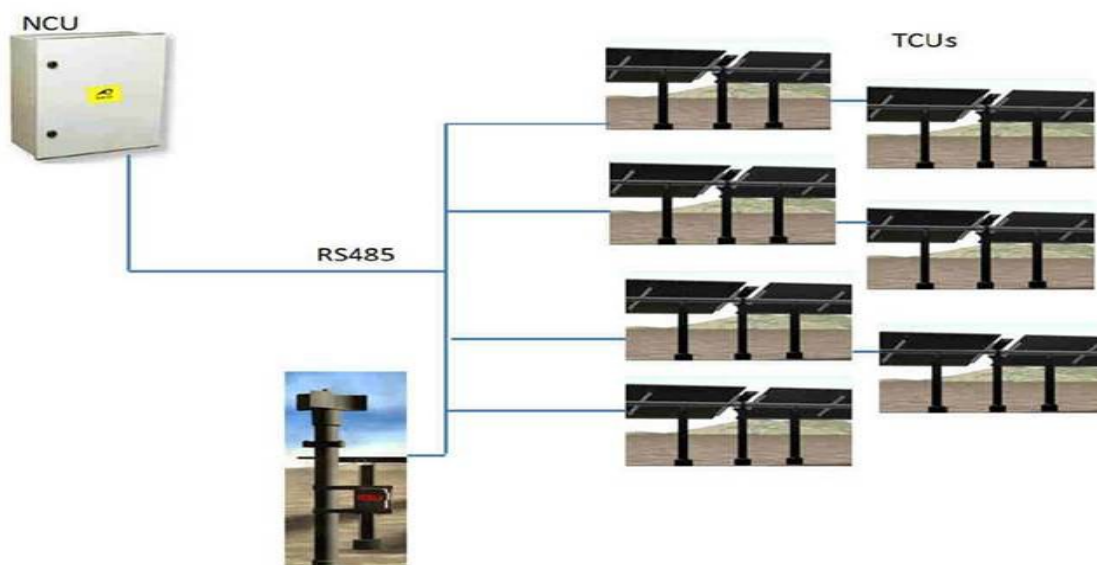
Imagen 10. Estación básica (NCU = Network Control Unit)
