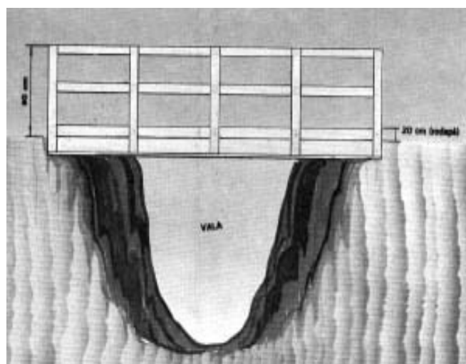
Figura 25: Pasarelas sobre zanjas.
