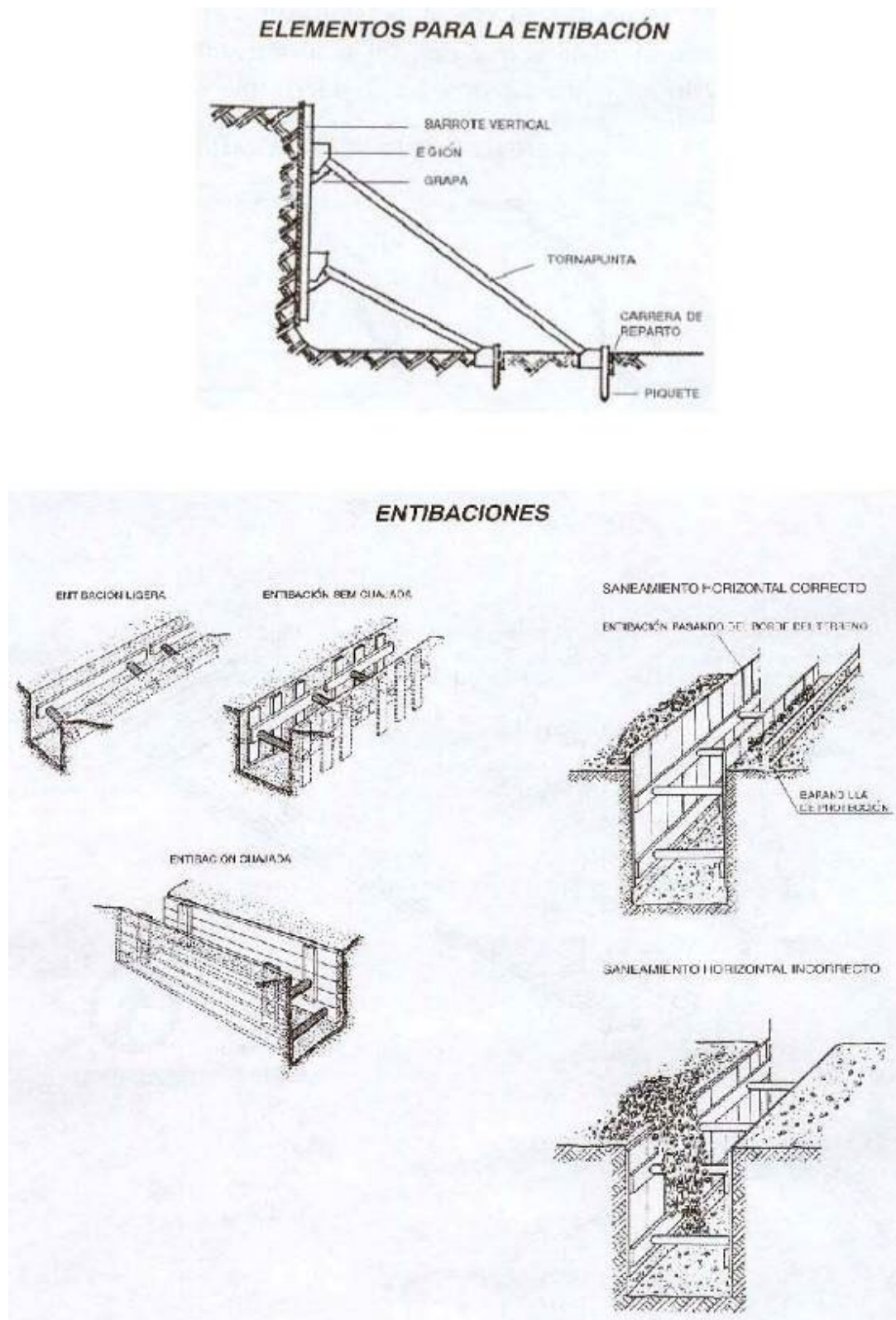
Figura 22: Protección, señalización y entibación de zanjas.
