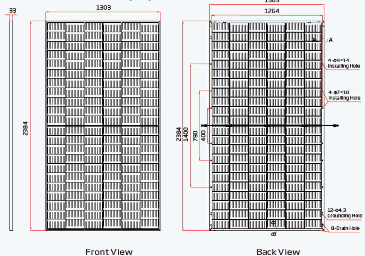
Imagen 2. Dimensiones físicas del módulo.
