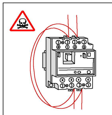
PUENTEADO DE ELEMENTOS DE PROTECCION.
