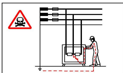
DEFECTOS DE AISLAMIENTO EN MAQUINAS SIN PROTECCION.
