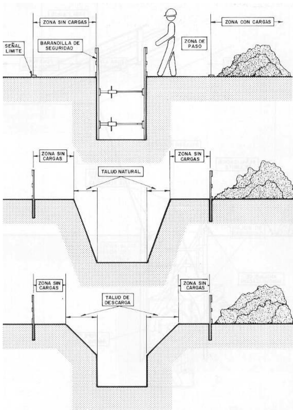
20: Protección, señalización y entibación de zanjas.
