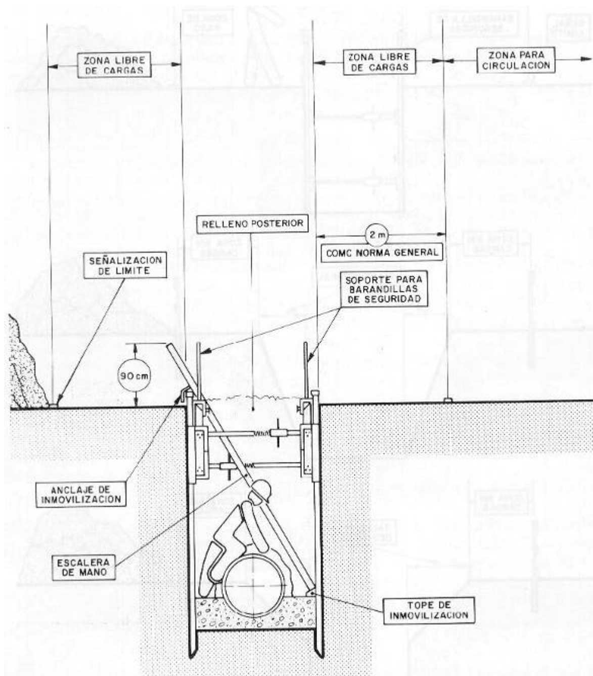
Figura 19: Protección, señalización y entibación de zanjas.
