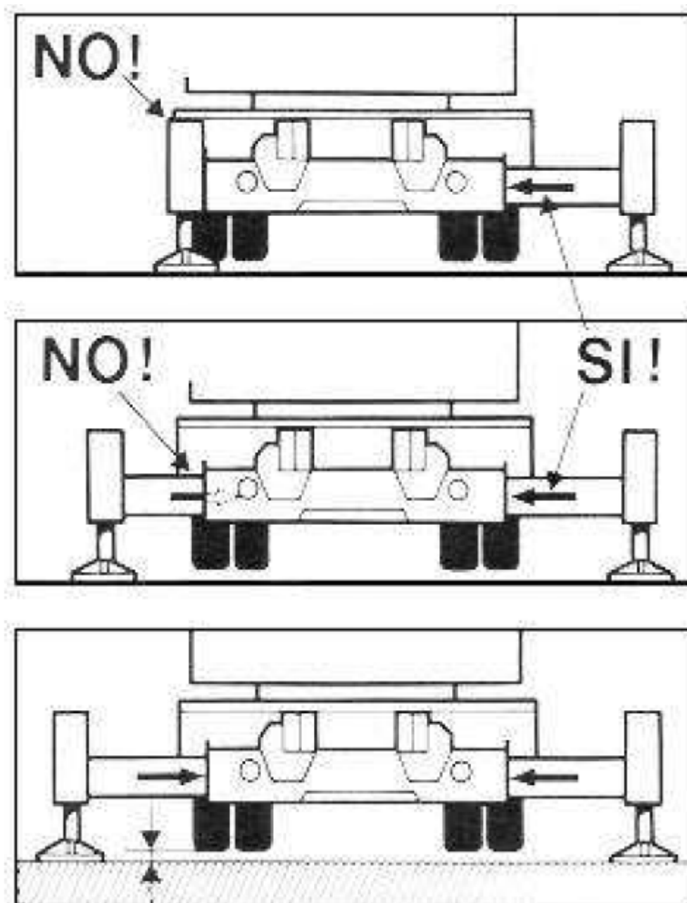
Figura 29: Estabilización de grúas.
