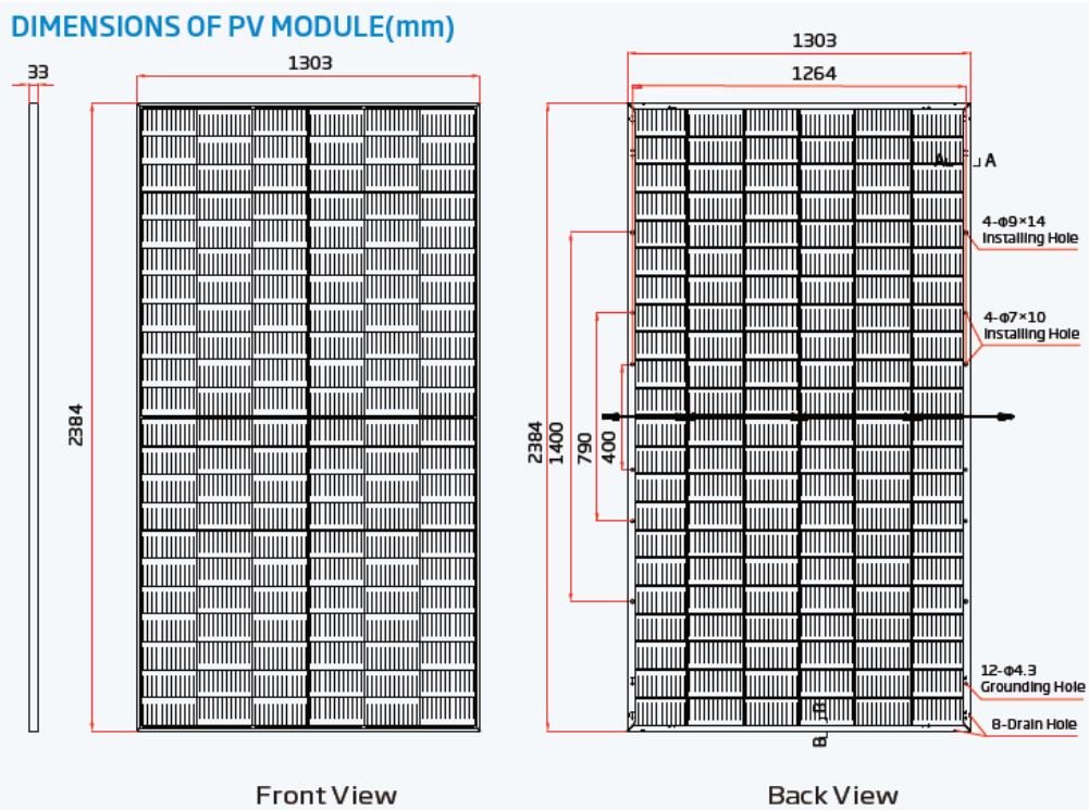
Imagen 1. Dimensiones físicas del módulo.
