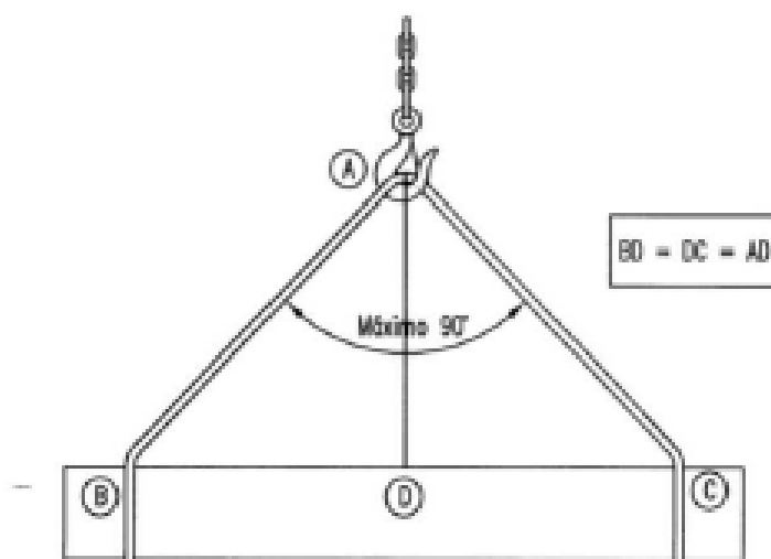
Figura 14: Ángulos de eslingado.
