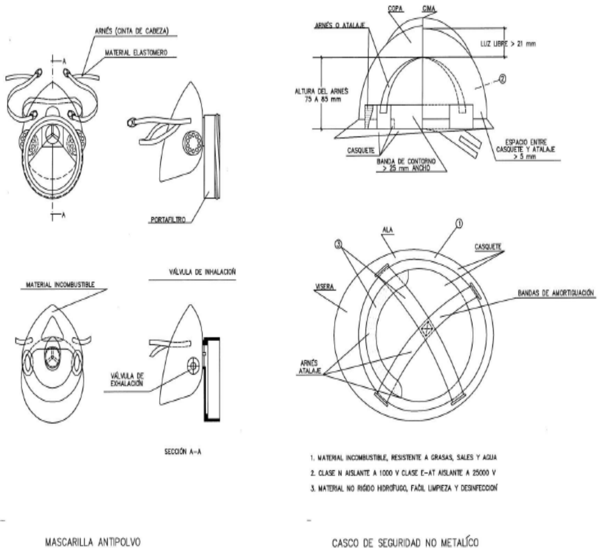
Figura 1: Mascarilla anti polvo y casco de seguridad.
