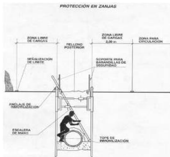
Figura 21: Protección, señalización y entibación de zanjas.
