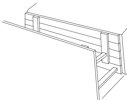
Figura 24: Protección, señalización y entibación de zanjas.
