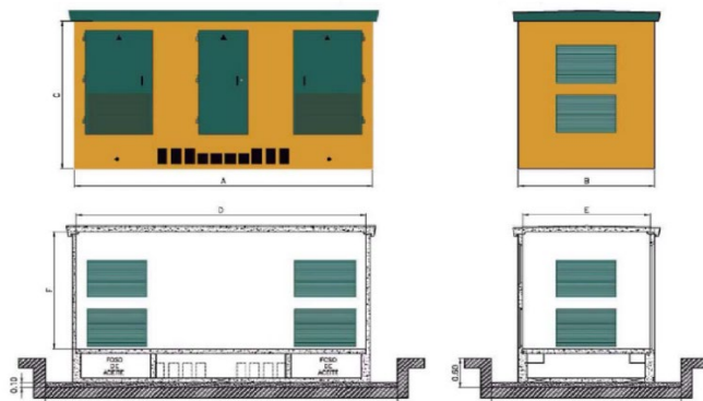
Imagen 7. Centro de Transformación.
