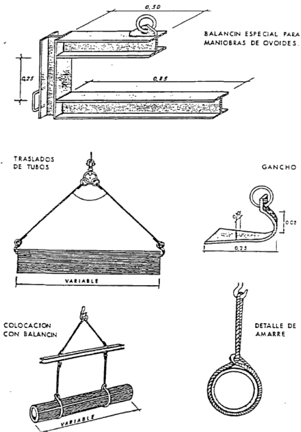
Figura 15: Útiles de izado.
