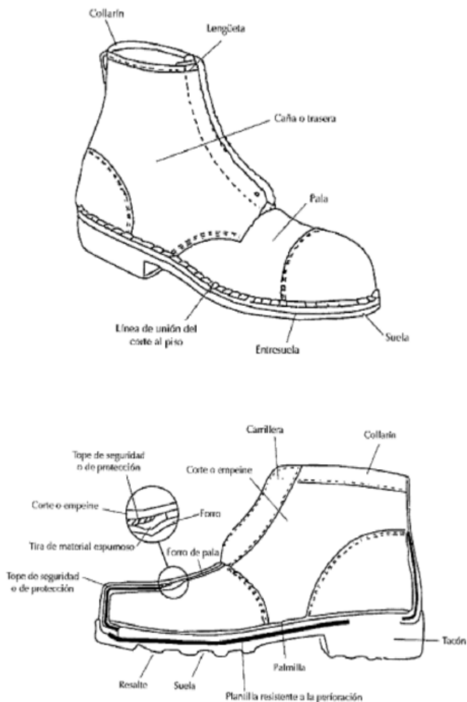
Figura 2: Calzado de seguridad.
