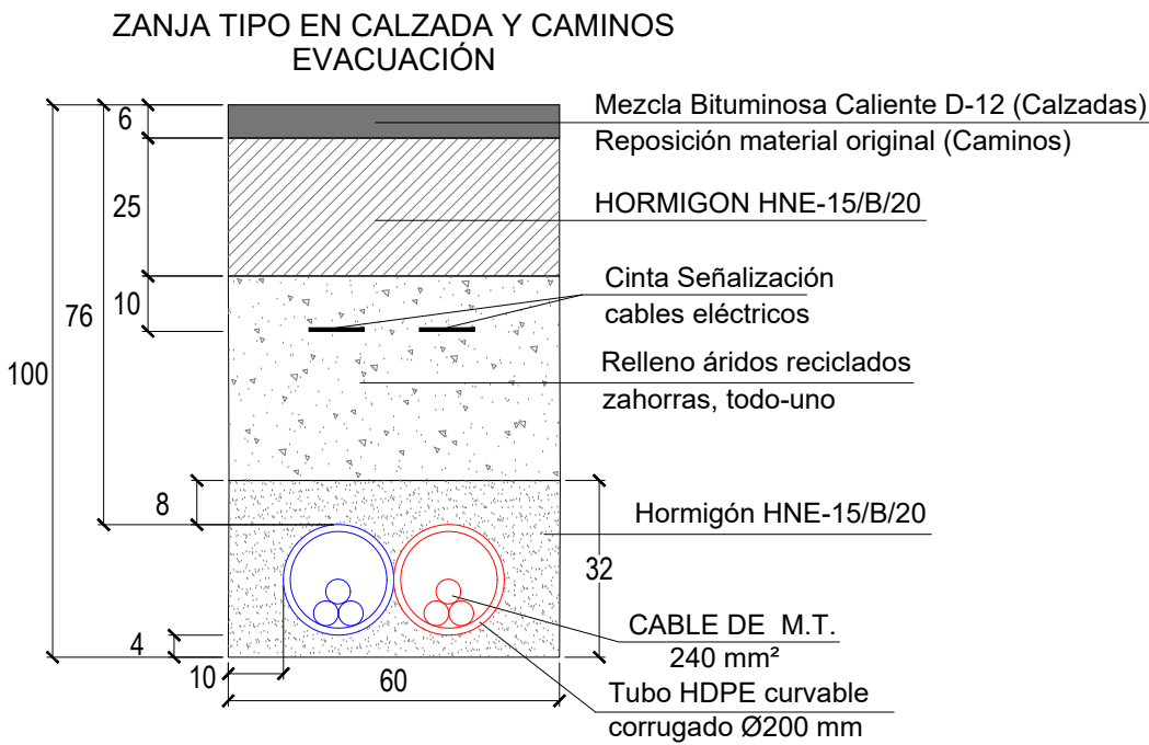
CANALIZACIÓN ENTUBADA 2 TUBO Ø200 NOTA: todas las cotas en centímetros ESCALA 1: 1/15
