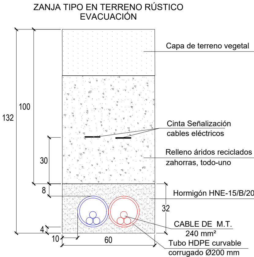
CANALIZACIÓN ENTUBADA 2 TUBO Ø200 NOTA: todas las cotas en centímetros ESCALA 1: 1/15
