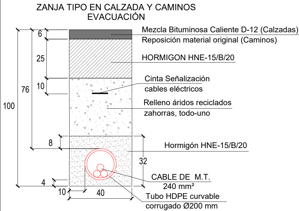
CANALIZACIÓN ENTUBADA 1 TUBO Ø200 NOTA: todas las cotas en centímetros ESCALA 1: 1/15
