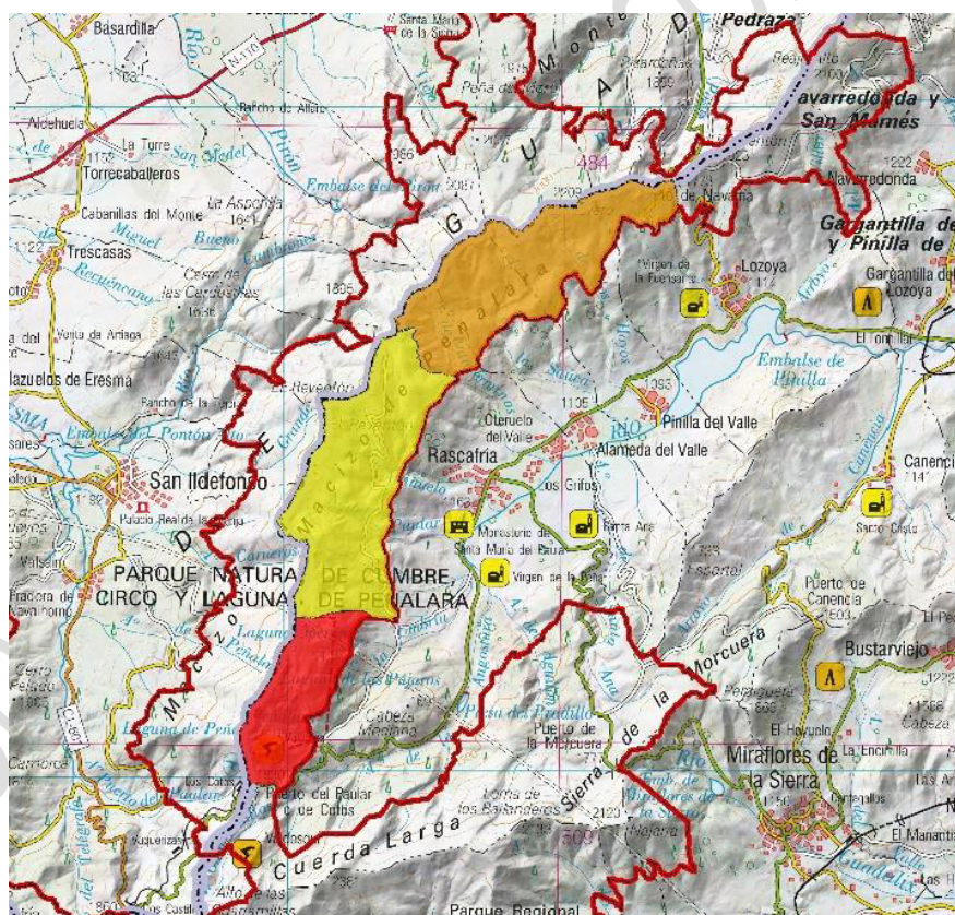
Figura 2. Sectores de clasificación Zona A1. Se identifican el Sector I, Sector II y Sector III.
