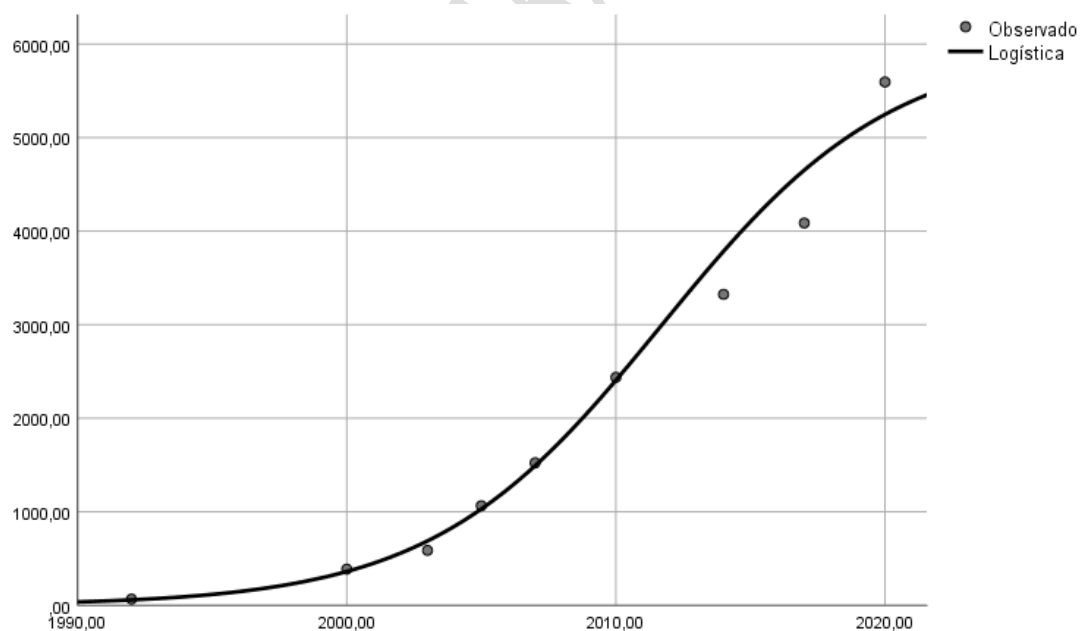
Figura 1. Evolución de la población de cabra montés en la zona de la Cuerda Larga-Pedriz desde el año de la introducción hasta la actualidad, a través del modelo de crecimiento logístico.
