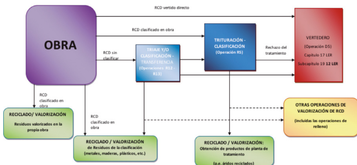
Figura 5. Esquema de gestión de RCD.
