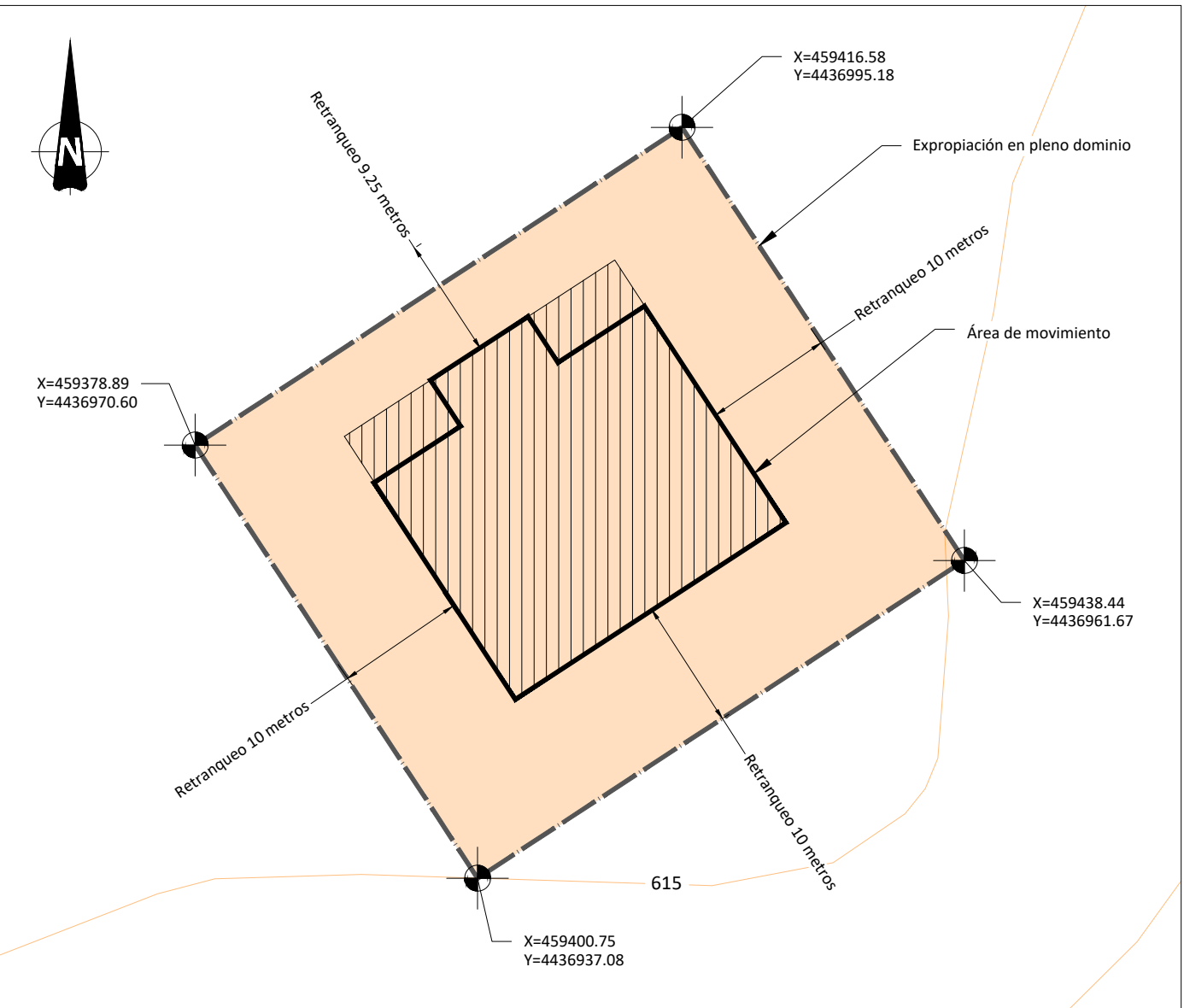
NUEVO DEPÓSITO DE REGULACIÓN- URBANIZACIÓN ZONA 2
