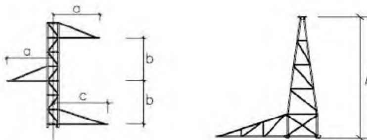
TIPO S Cúpula
