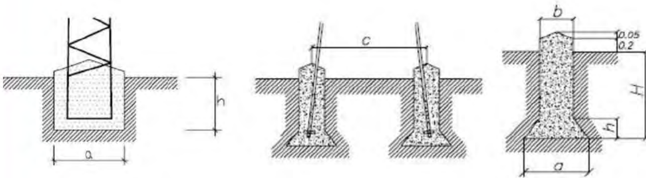
Cimentación monobloque Cimentación tetrabloque cuadrada o circular con cueva
