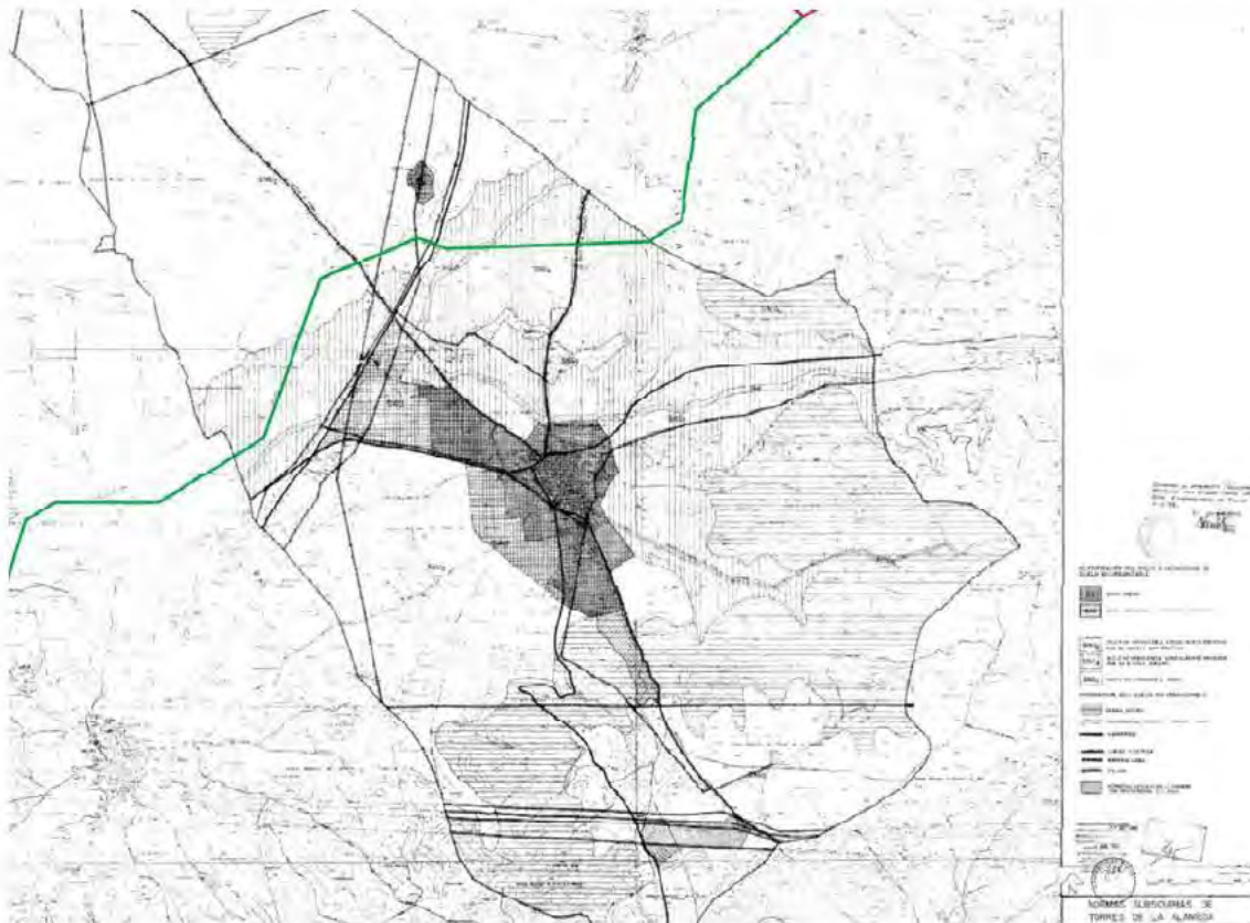
Ilustración 22: Trazado del tramo en simple circuito de RT1 sobre el planeamiento urbanístico del término municipal de Torres de la Alameda.
