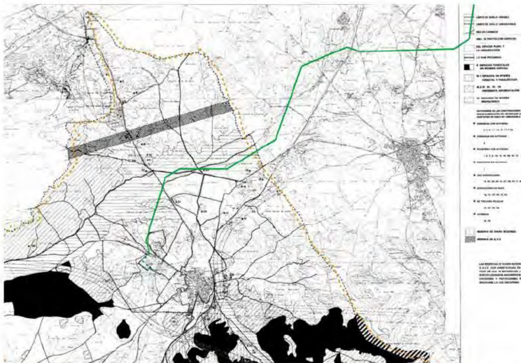
Ilustración 23: Trazado del tramo en simple circuito de RT1 sobre el planeamiento urbanístico del término municipal de Loeches.
