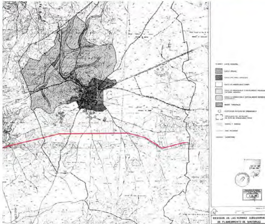
Ilustración 18: Trazado del tramo en doble circuito RT1 y RD2 sobre el planeamiento urbanístico del término municipal de Santorcaz.
