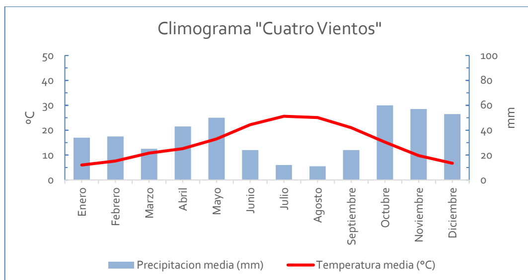
Figura 3.4. Climograma para la estación de Cuatro Vientos. Fuente: Elaboración propia.
