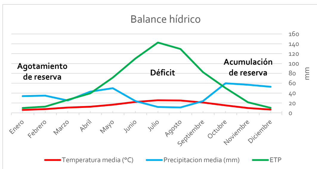
Figura 3.4.1. Balance hídrico para la estación de Cuatro Vientos. Fuente: Elaboración propia.
