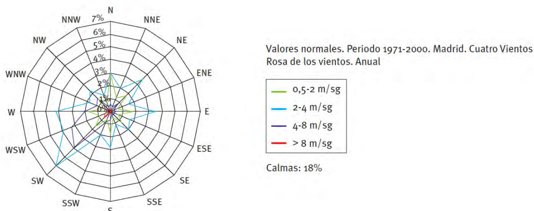
Figura 3.4.2. Rosa de los vientos obtenida de los valores normales de viento para el periodo 1971-2000 en la estación meteorológica de Madrid (Cuatro Vientos). Fuente: IDAE.
