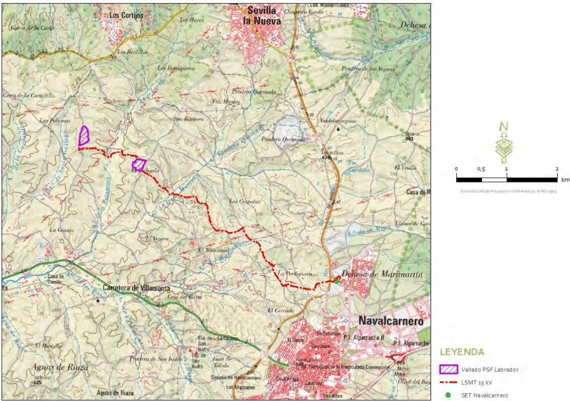
Figura 1.3.1.a. Localización de la Planta Solar Fotovoltaica Labrador e infraestructuras de evacuación. Fuente: Proyecto ejecutivo de la Planta Solar Fotovoltaica Labrador.
