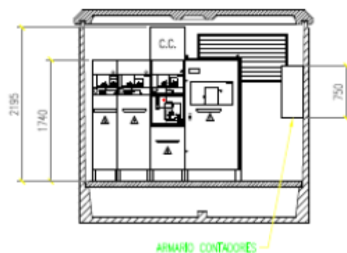
Figura 6. Esquema Centro de Medida
