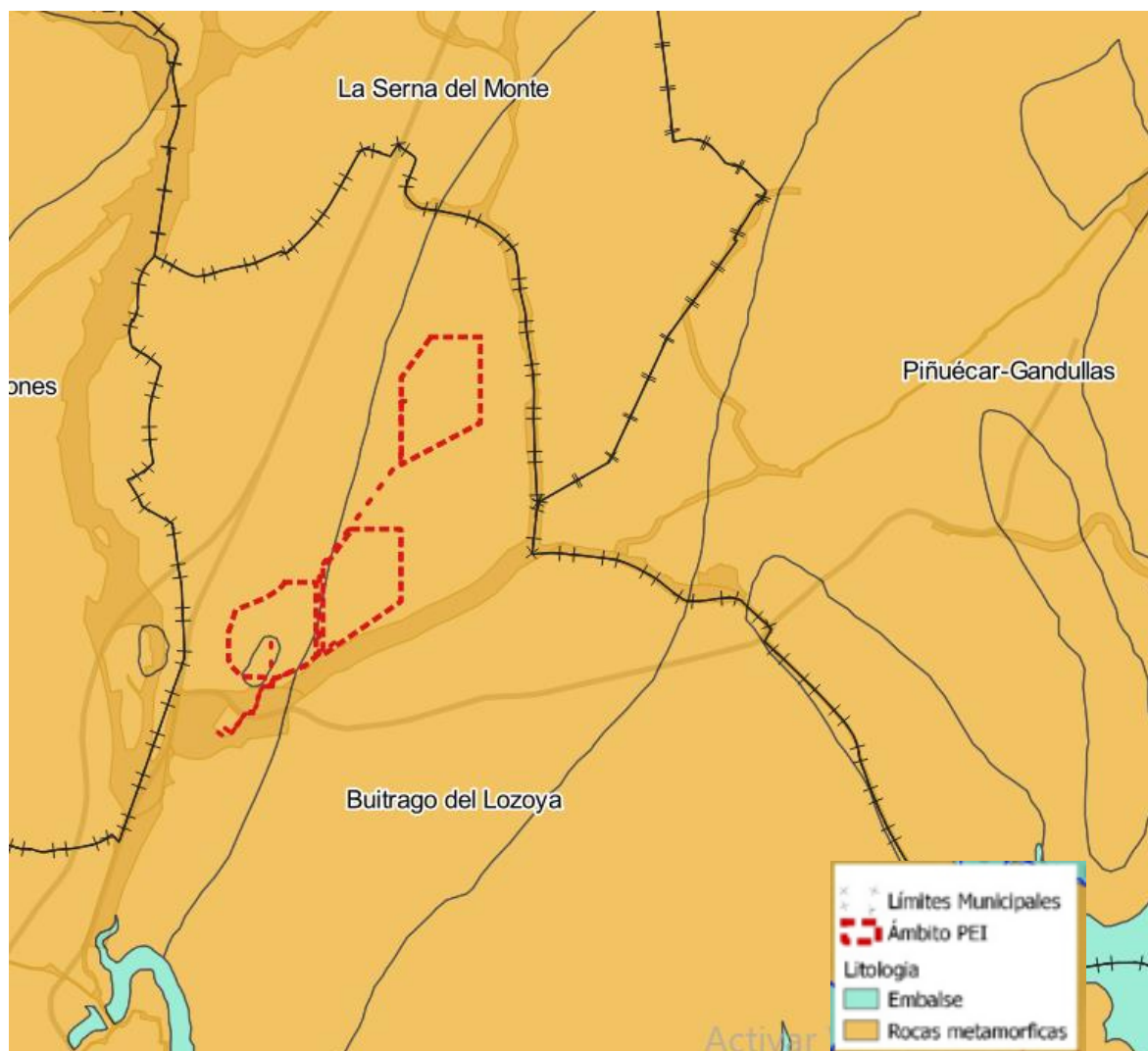
Fig. Mapa Litografico del ámbito de estudio. Fuente: IDE Comunidad de Madrid. Elaboración propia
