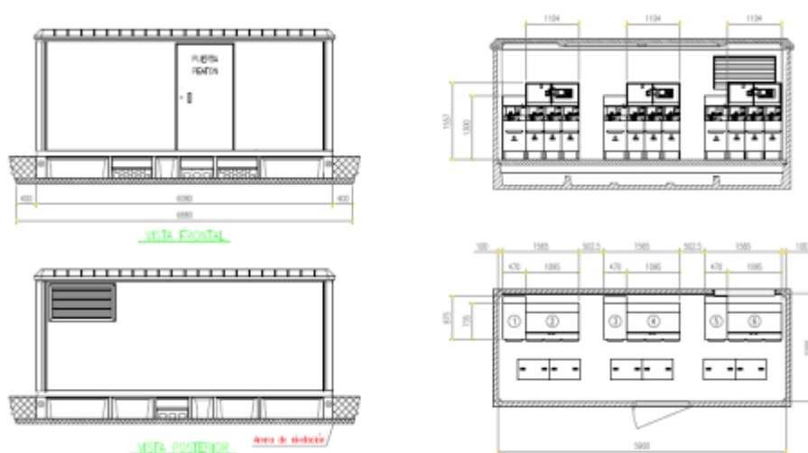
Figura 10. Esquema Centro de Seccionamiento
