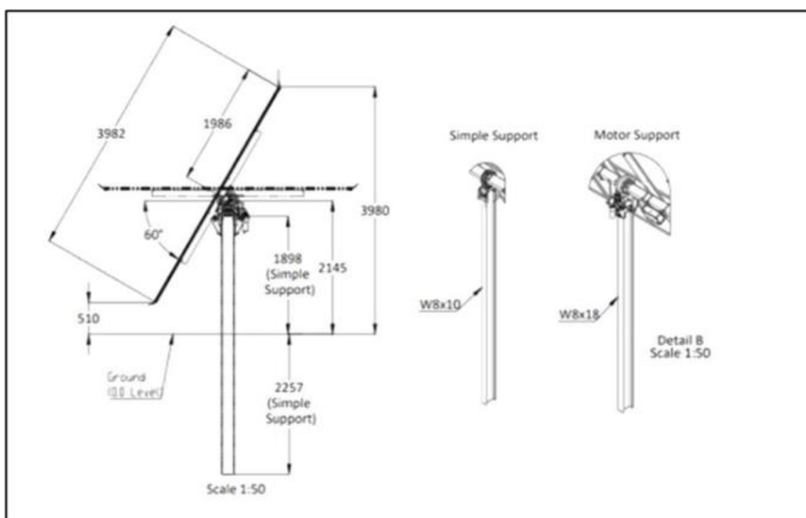
Plano de las dimensiones del tracker.
