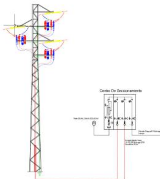
Figura 13. Esquema conversión aéreo-subterráneo
