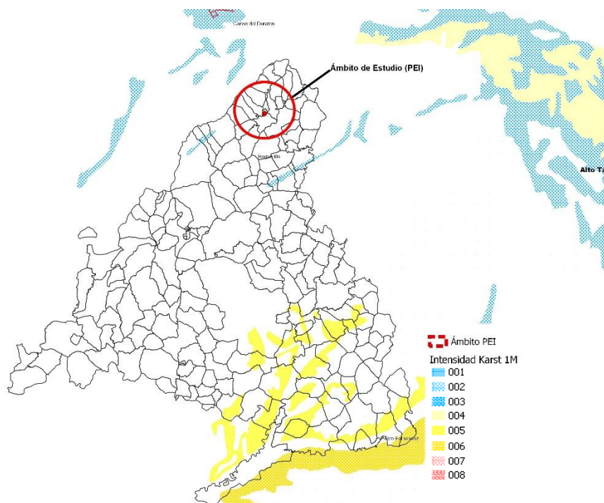
Mapa de Peligrosidad Karst. Fuente: IGME
