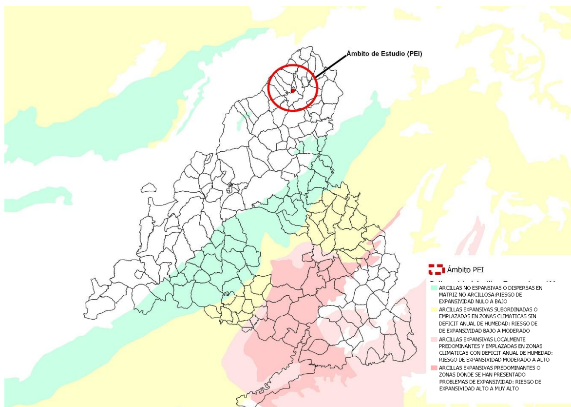
Mapa de Peligrosidad Arcillas Expansivas. Fuente: IGME
