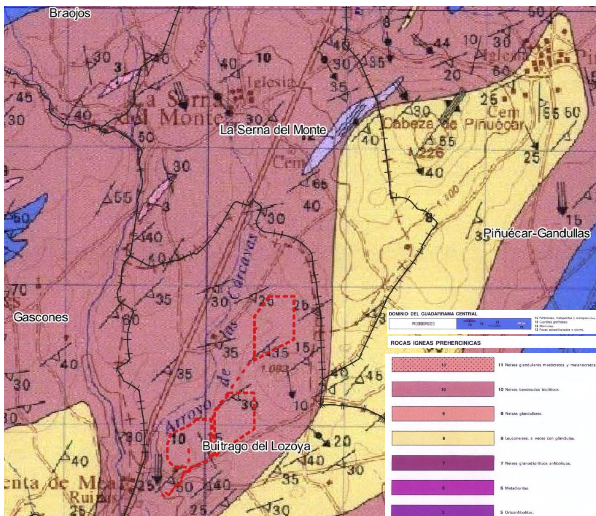
Mapa Geológico del ámbito de estudio. Fuente: Mapa Geológico Continuo de España a escala 1/50.000.
