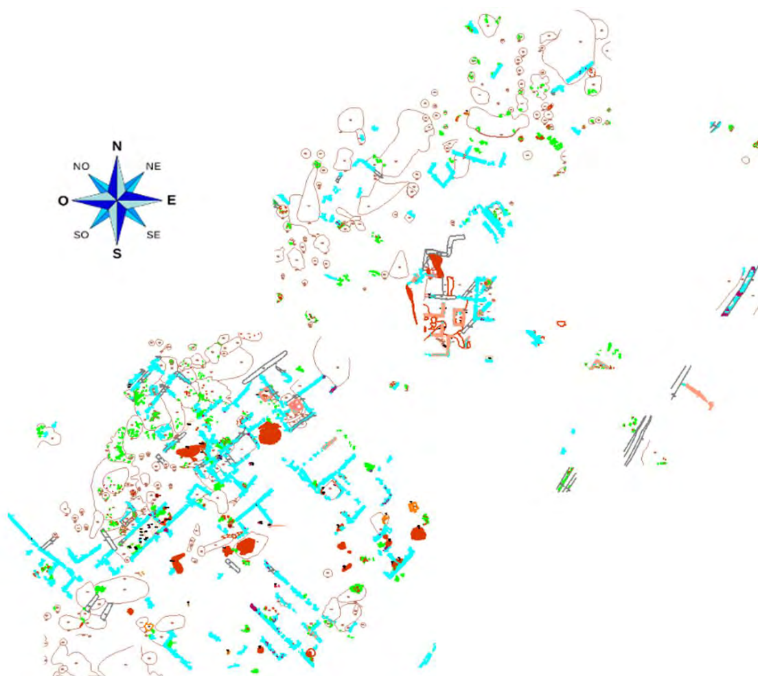
Planta de las estructuras del Vicus Altoimperial Ermita de Santiago..
