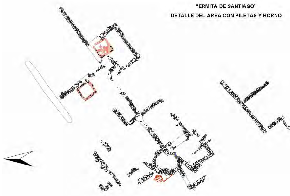
Localización de piletas para decantación de vino y/o aceite.
