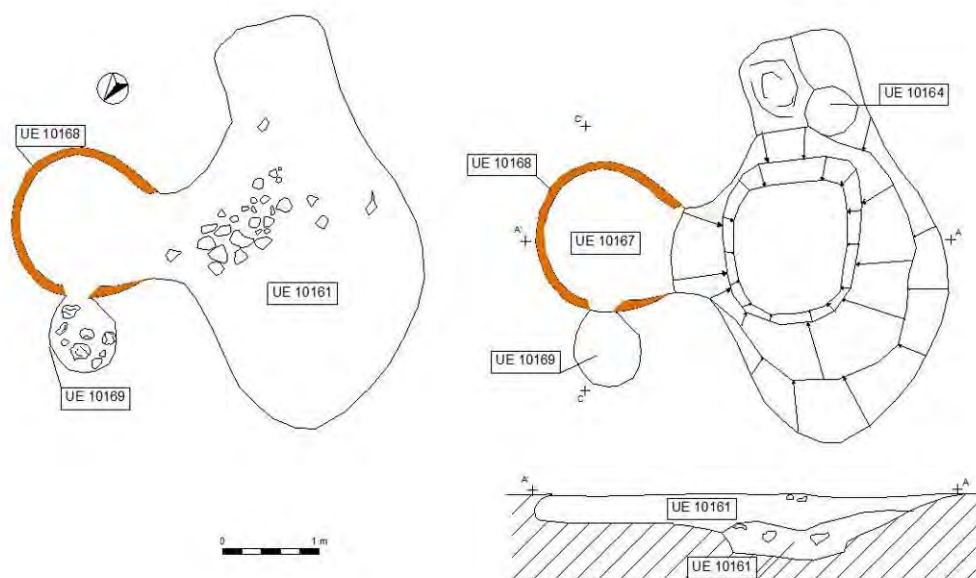
Proceso de excavación del horno C-10160
