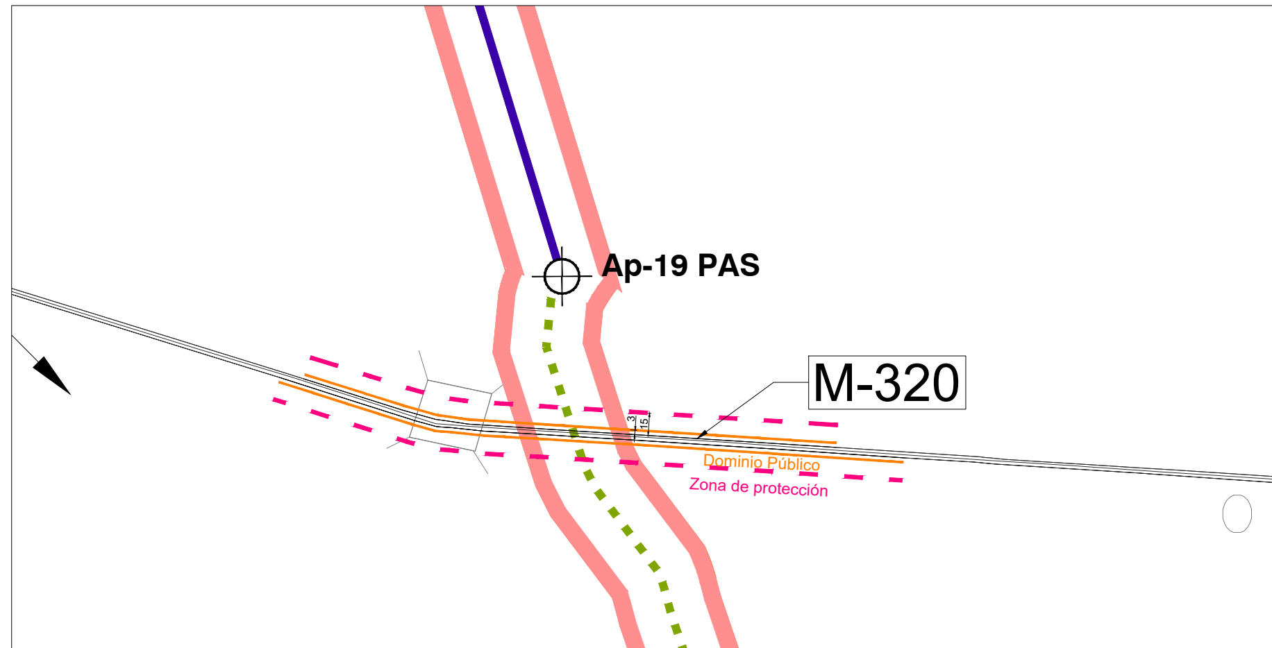
DETALLE A
