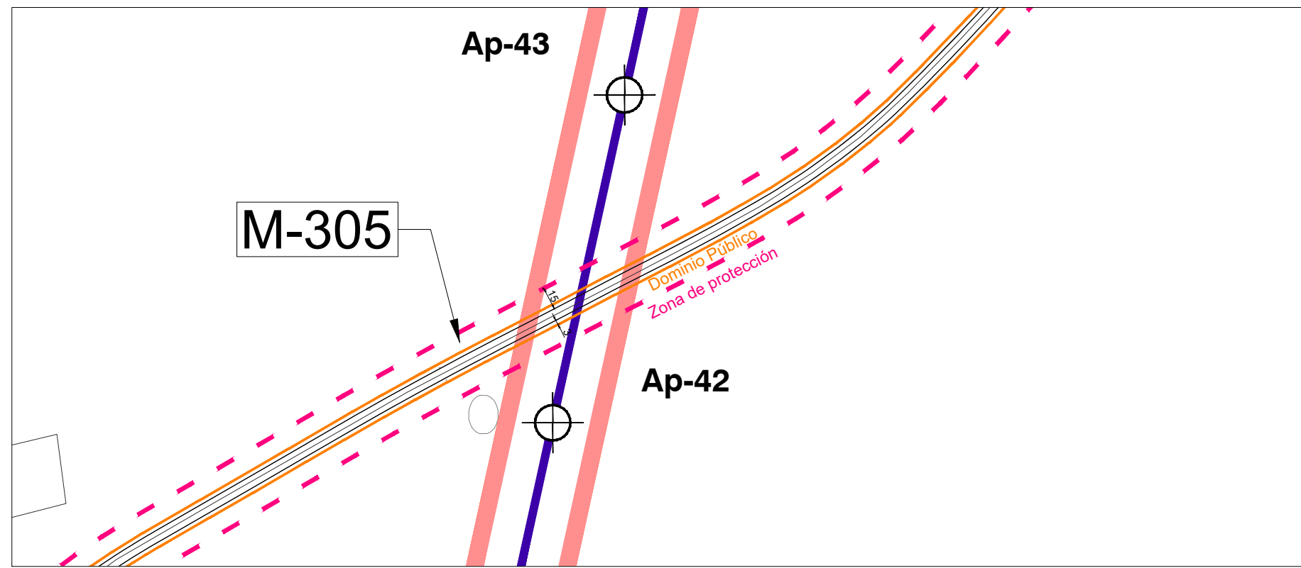
DETALLE C
