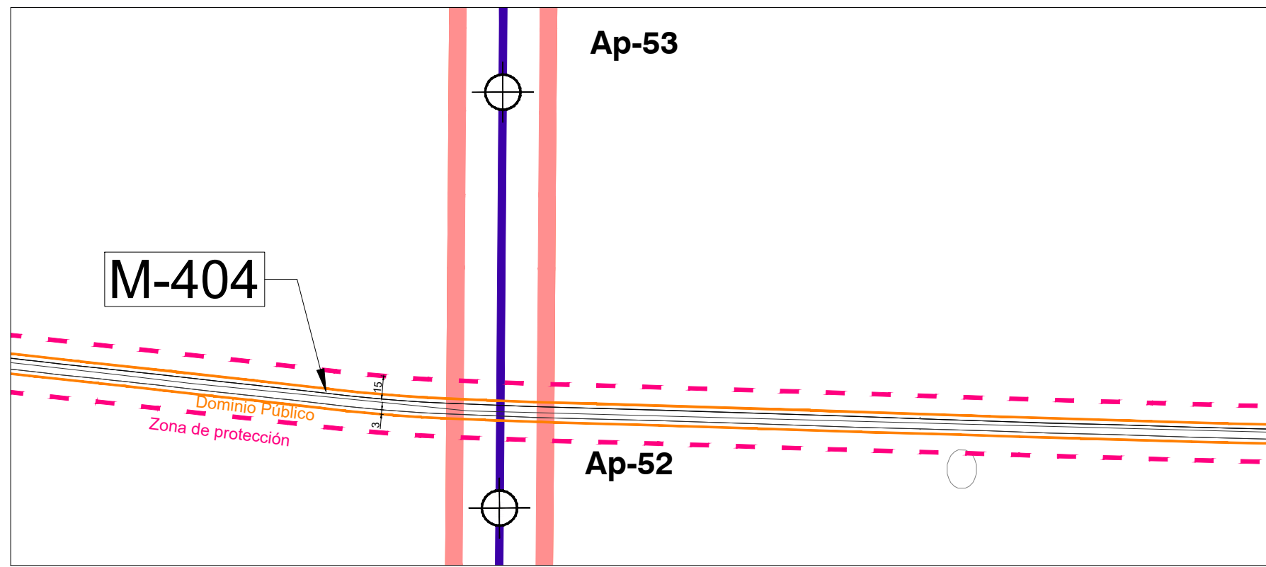
DETALLE F
