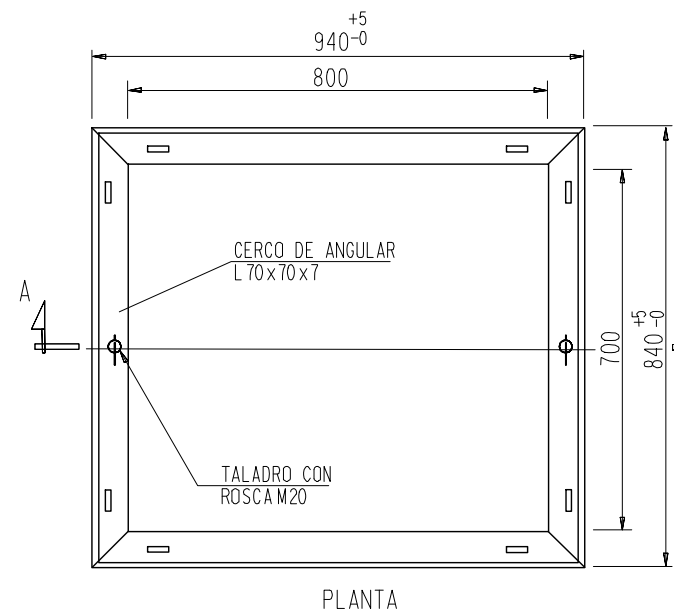
DETALLE 1 SOPORTE DE ENGANCHE DE POLEAS CERCO
