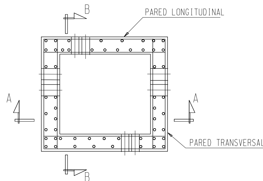
SECCION C-C
